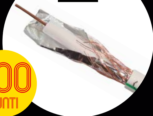
SAT703B CONDUTTORE INTERNO IN RAME ROSSO (CU) Ø 1,13 MM (400+100 e multipli)
